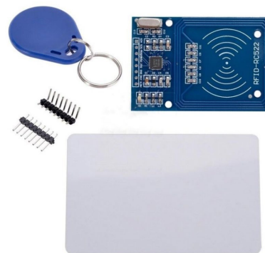
RFID 感應模組
