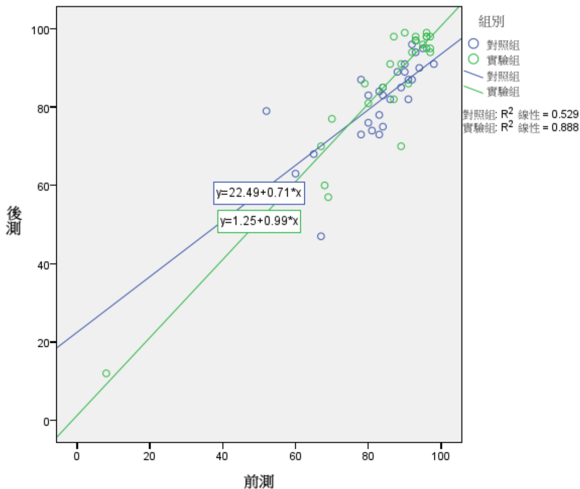
圖一 實驗組與對照組所建構之迴歸方程式
