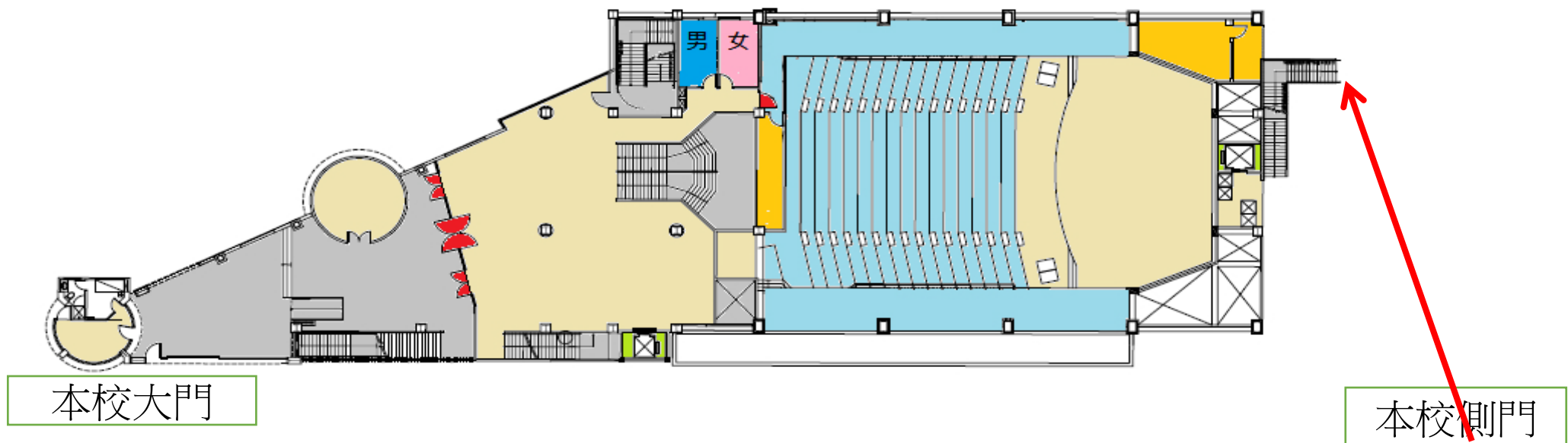
三重區碧華國小活動中心平面圖1F
